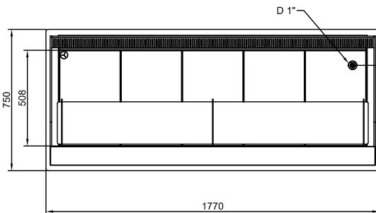
Boven aanzicht
