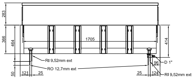
Zij aanzicht
